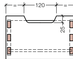
Ausfräsung: C
