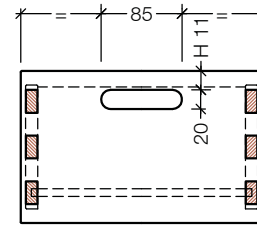
Ausfräsung: A
