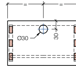
Ausfräsung: B
