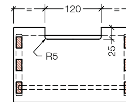
Ausfräsung: F
