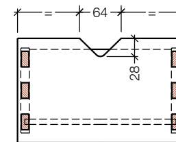
Ausfräsung: D
