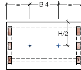
Griffbohrungen
